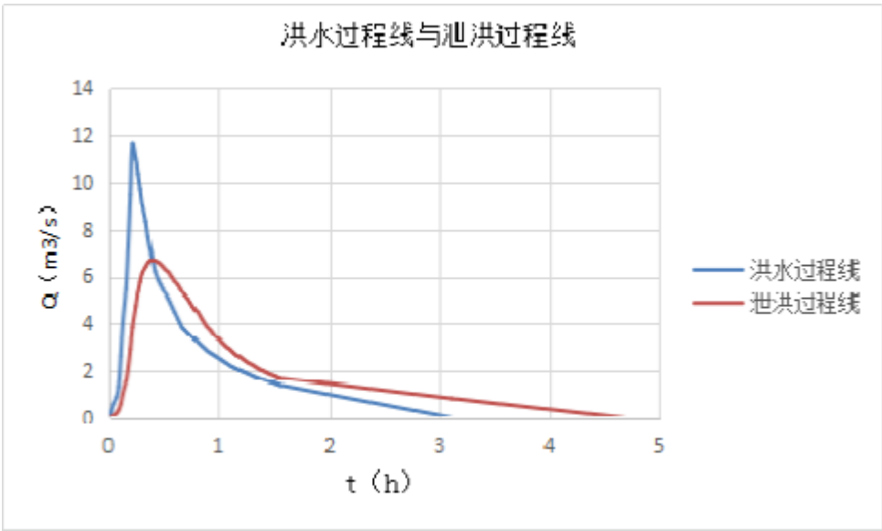
图 5-8 洪水过程线与泄洪过程线
