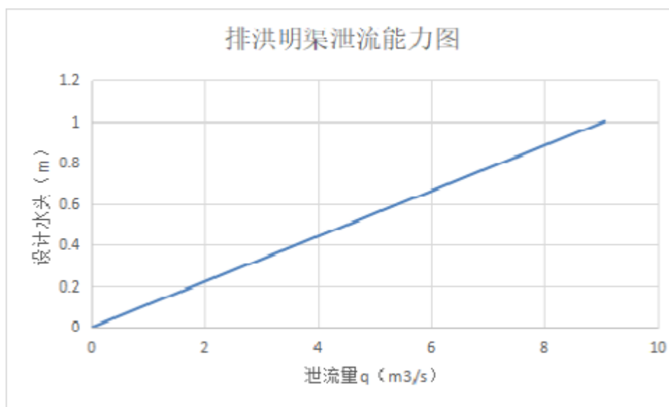
图 5-5 排洪明渠泄流能力图
