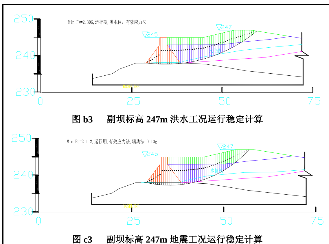
图 5-2 坝体稳定性计算结果
