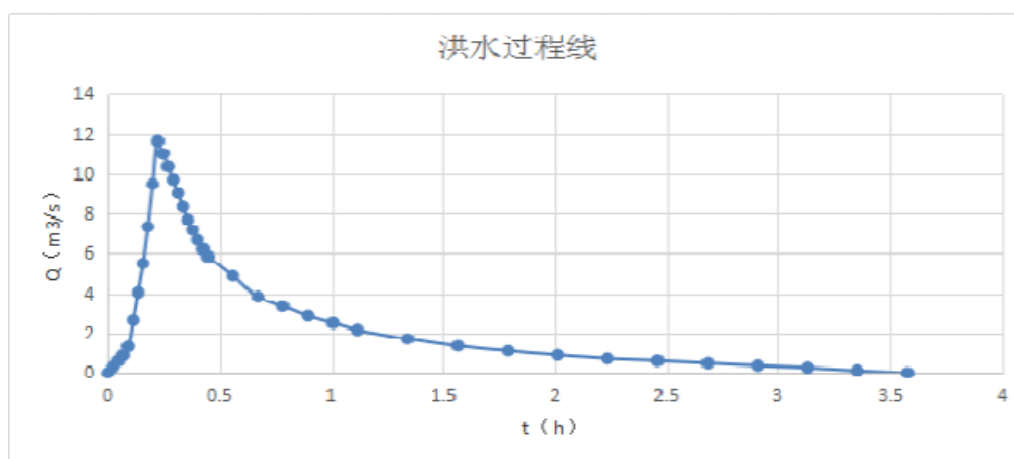
图 5-3 洪水过程线
