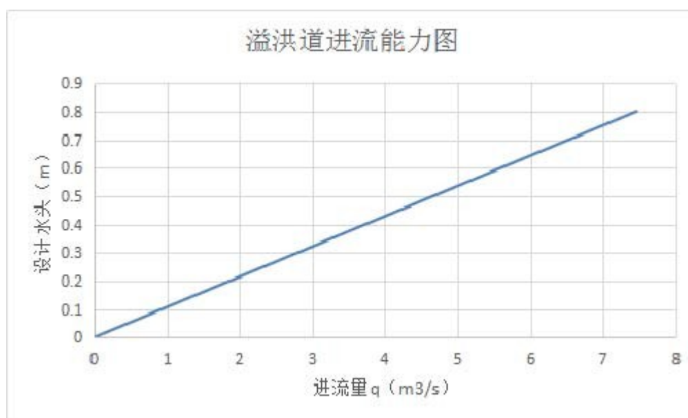
图 5-4 溢洪道进流能力图
