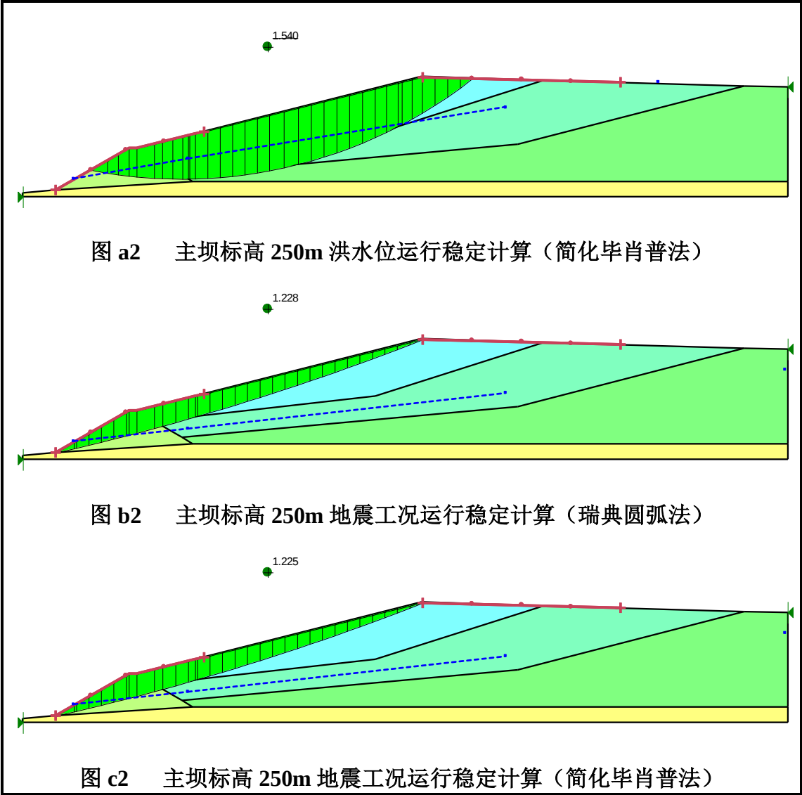
图 5-1 坝体稳定性计算结果
