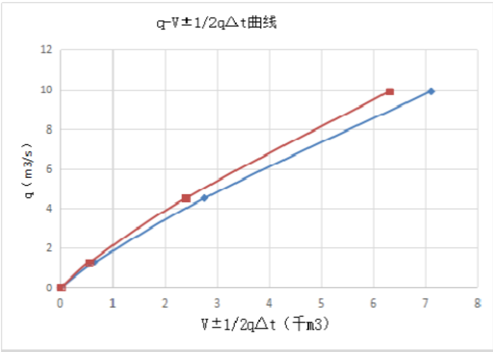
图 5-7 V\pm 1/2q\Delta t\sim q 曲线图
