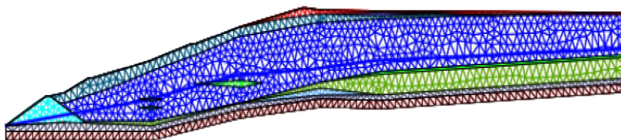
图 2-2 坝体现状浸润线图
