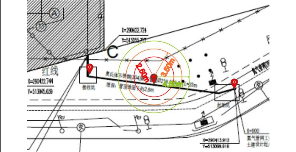
事故后果
